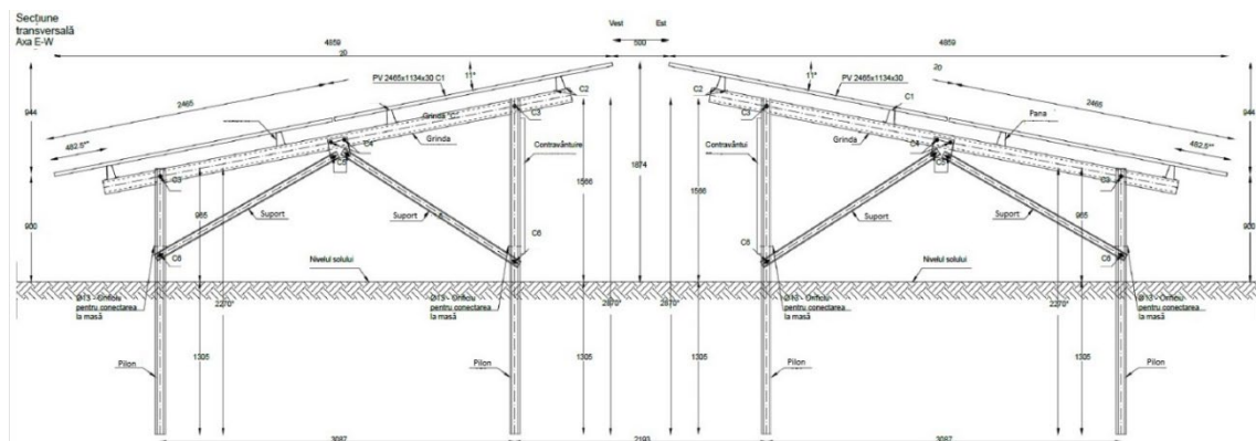
Figura 1. Desen indicativ - Detalii structură – secțiune transversală
